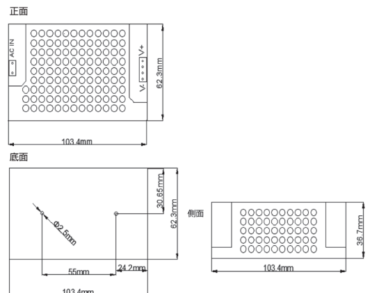
外形図
