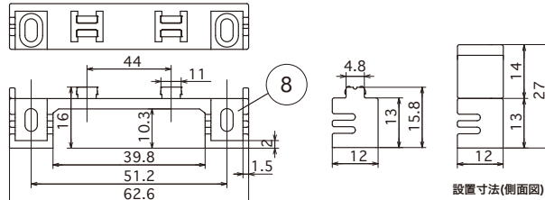
設置寸法(側面図)
