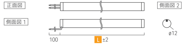
片端リード線・コネクタ仕様
