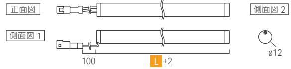
片端リード線・コネクタ仕様
