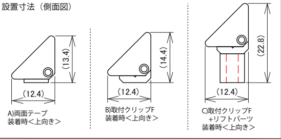
設置寸法 (側面図)
