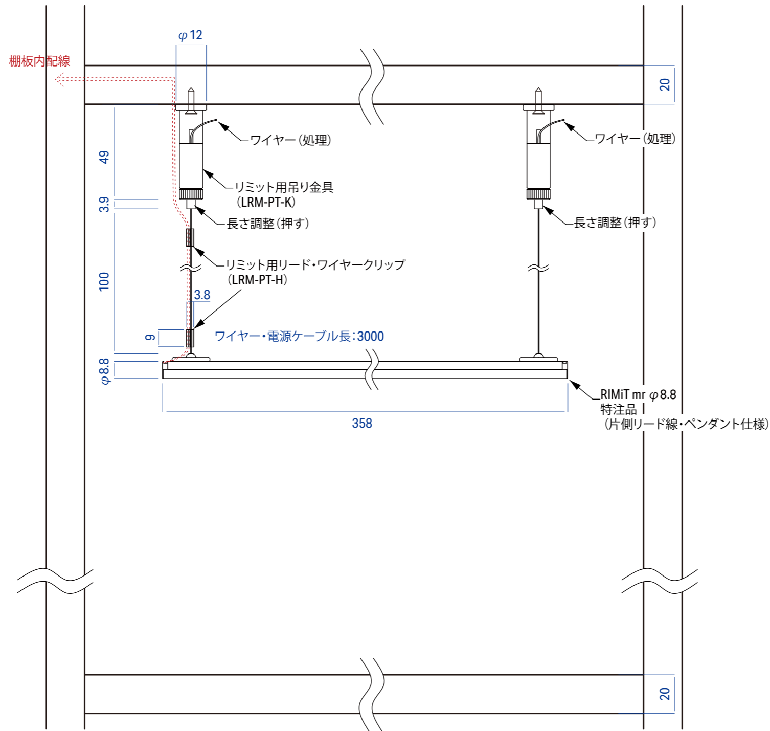
断面詳細図 S=1:2
