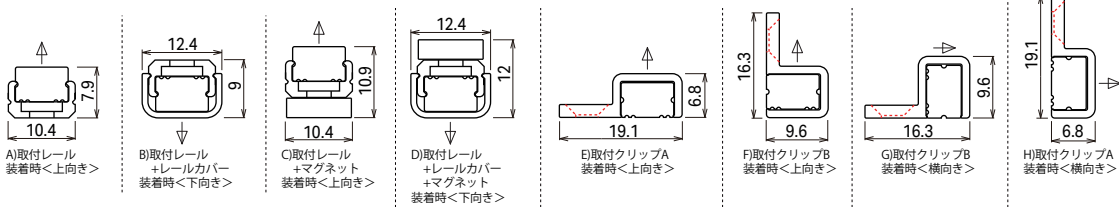
設置寸法（側面図）
