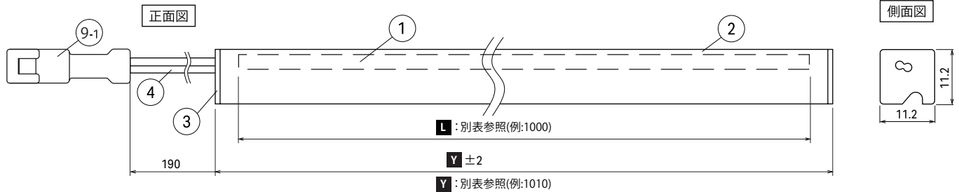
設置寸法（側面図）
