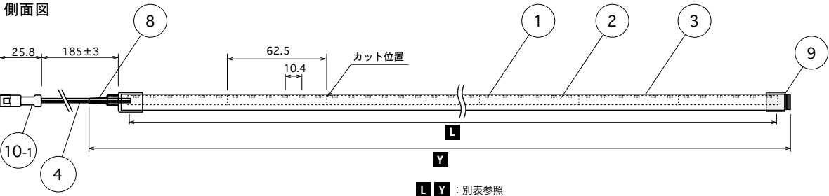
側面図
