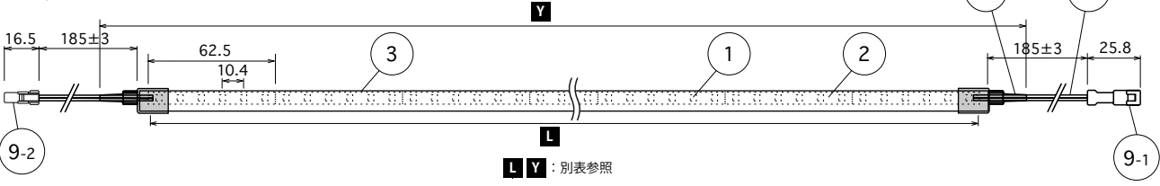
正面図
