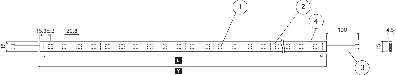
正面図
