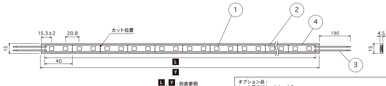
正面图
