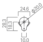
側面図 2
