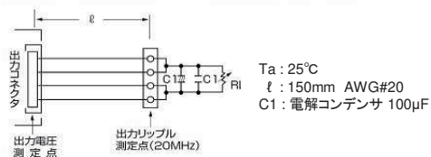
図 1 : 出力電圧および出力リップル電圧測定方法
