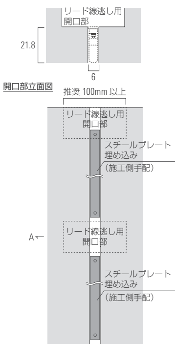
断面図A (灯具無)
