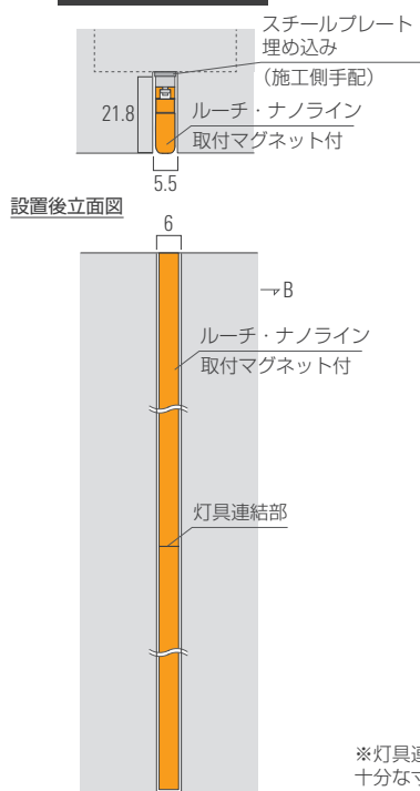
断面図B (灯具有)
