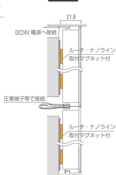
断面図C
